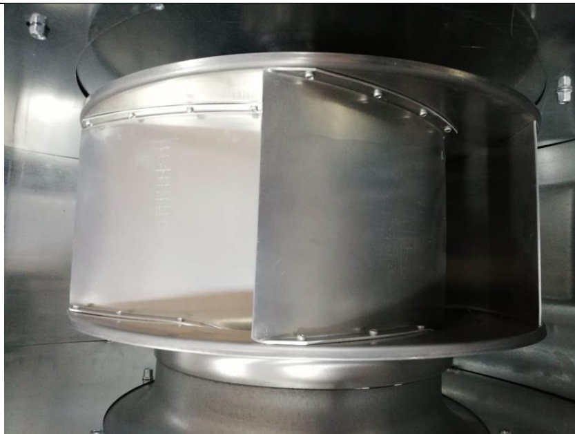
Photo 4. Fan
